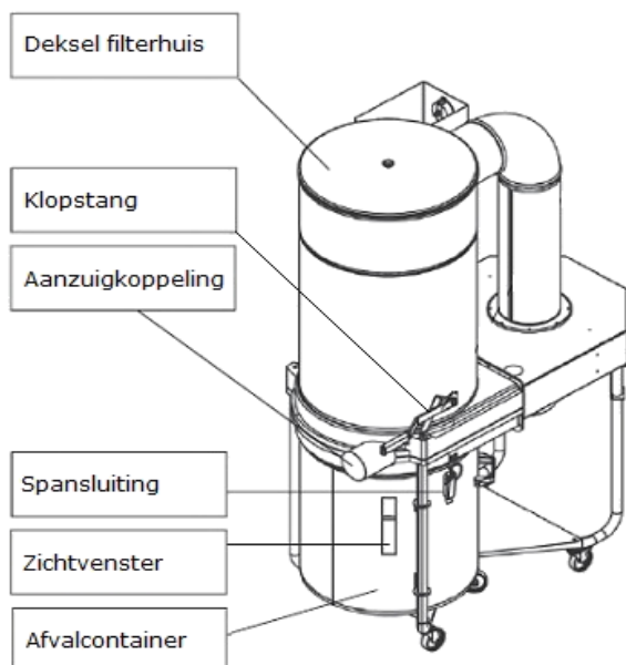
Achterzijde stofafzuiger
