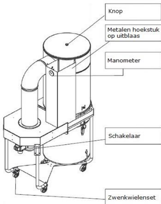
Voorzijde stofafzuiger
